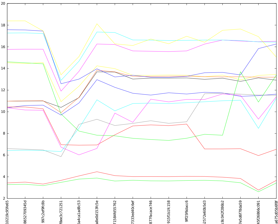
penryn-sse4-sgemmm
